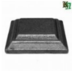
Основание баясины, арт. 13.314 80х80х20мм, без отв. Вес: 0.285 кг Цена: 115 руб.
