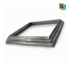
Основание блясины, арт. 13.310.02 122x122x1мм, кв.100x100мм Вес: 0.06 кг Цена (за шт): 48 руб.
