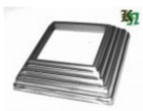
Основание блясины, арт. 13.310.01 142x142x1мм, кв.100x100мм Вес: 0.135 кг Цена: 70 руб.
