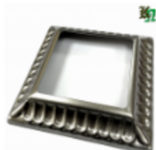
Основание блясины штампованное, арт. 8.879 170x170x1 кв. 100x100 Вес: 0.19 кг Цена (за шт): 150 руб.
