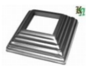
Основание блясины, арт. 13.380.02 122x122x1мм, кв.80x80мм Вес: 0.1 кг Цена: 41,90 руб.
