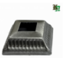
Основание балясины, арт. 8.6020 60x60x1мм, кв.20x20мм Вес: 0.04 кг Цена (за шт): 38,50 руб.
