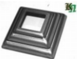
Основание балясины, арт. 13.329.01 44x44x1мм, кв.17x17мм Вес: 0.021 кг Цена: 20 руб.
