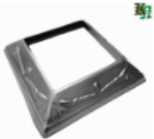
Стальное, штампованное декоративное основание., арт. 8.899 200x200x1мм кв.120x120 Вес: 0.22 кг Цена (за шт): 240 руб.
