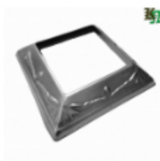
Стальное, штампованное декоративное основание., арт. 8.899 200х200х1мм кв.120х120 Вес: 0.22 кг Цена (за шт): 240 руб.
