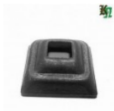
Основание балясины, арт. 7.324 50x50мм, кв.16x16мм Вес: 0.07 кг Цена: 49 руб.
