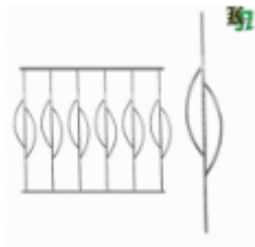
Балясина с центральной частью "торсион", арт. 3092 1000x165мм, кв.12x12мм Вес: 2.12 кг Цена (за шт): 350 руб.
