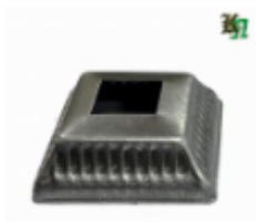
Основание балясины, арт. 8.6020 60x60x1мм, кв.20x20мм Вес: 0.04 кг Цена (за шт): 38,50 руб.
