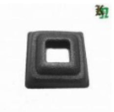
Основание баясины, арт. 7.327 40х40мм, кв.12х12мм Вес: 0.04 кг нет в наличии
