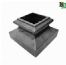
Вставка в балясину, арт. 277.30 70x43мм, на кв.30x30мм Вес: 0.45 кг Цена: 150 руб.
