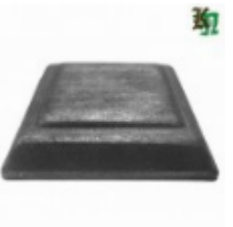
Основание баясины, арт. 7.310 100х100х20мм, без отв. Вес: 0.27 кг Цена: 150 руб.
