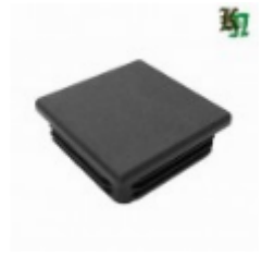
Заглушка пластиковая, арт. 35.30 кв.30x30мм Вес: 0.006 кг Цена: 10 руб.
