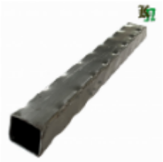
Труба профильная, арт. 40402Т 3000x40x40мм Вес: 7.2 кг Цена (за штуку): 850 руб.
