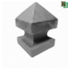
Наконечник, навершие, арт. 012GA 60x60 95x70мм, отв. кв.60x60мм Вес: 0.6 кг Цена: 208 руб.
