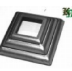
Основание баясины, арт. 13.327.01 44х44х1мм, кв.13,5х13,5мм Вес: 0.02 кг нет в наличии
