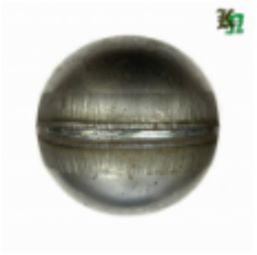
Шар пустотелый, арт. 7.100 д=80х1,5мм Вес: 0.18 кг Цена: 125 руб.
